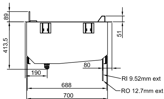
Zij aanzicht
